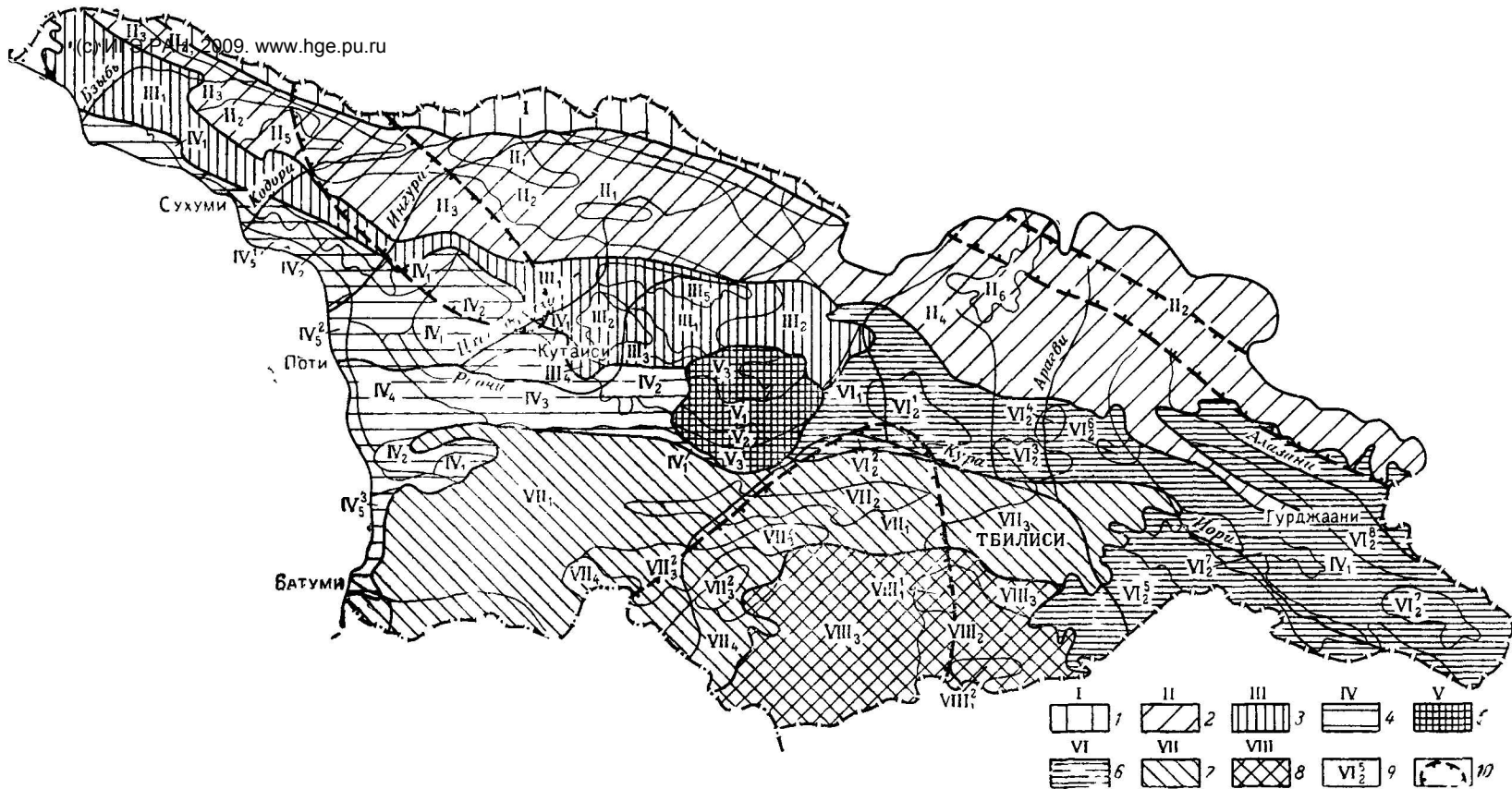
Рис. 46. Схема инженерно-геологического районирования территории Грузии (составили И. М. Буачидзе, К. И. Джанджгава, В. Ш. Чумбуридзе) 1—область кристаллического ядра осевой части антиклинория Большого Кавказа; 2—область высокогорья складчатой системы Южного склона Большого Кавказа; 3—область среднегорья западной части складчатой системы Южного склона Большого Кавказа; 4—область западного погружения Грузинской глыбы; 5—область Дзирульского кристаллического массива; 6—область восточного погружения Грузинской глыбы; 7—область Аджаро-Триалетской складчатой системы; 8—область Артвино-Болнисской (Сомхитской) глыбы; 8—районы и подрайоны (см. в тексте), 10—граница между 7- и 8-балльными сейсмическими зонами
