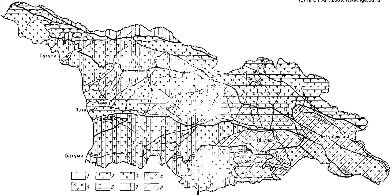
Рис. 24 Схематическая гидрохимическая карта грунтовых вод Грузии (составили О. П. Менгешавили, М. В. Мзареулишвили, Б. С. Мхеидзе, Г. И. Буачидзе)
