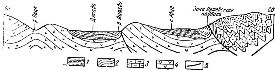
Рис. 21. Схематический гидрогеологический разрез района Джавского месторождения минеральных вод (составили В. Ш. Чумбуридзе и Д. Л. Юзбашев)
