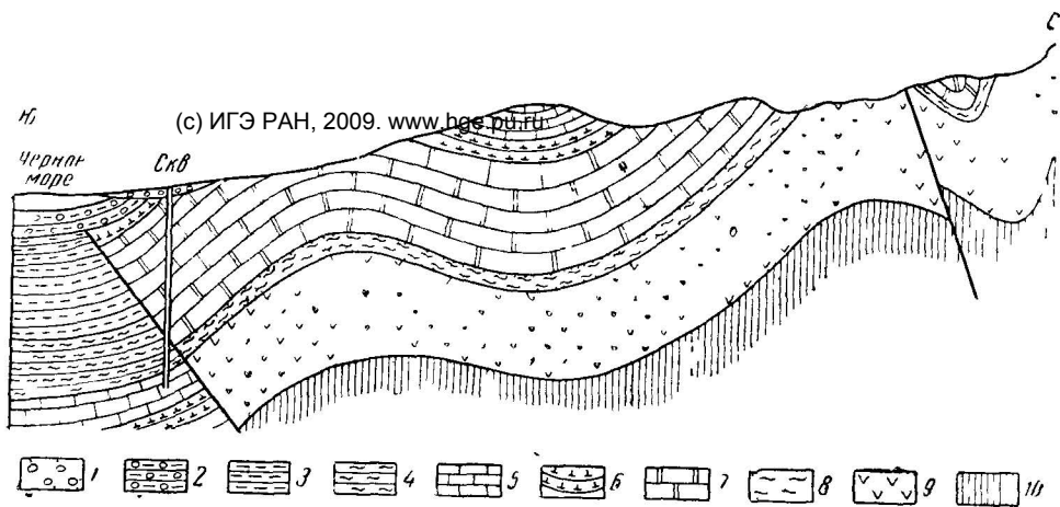
Рис. 20. Гидрогеологический разрез Гагрского массива (составил О. А. Шубладзе) 1 — водоносный горизонт средне- и древнечетвертичных отложений; 2 — водоносный горизонт отложений понт-мэотиса; 3 — спорадически обводненные отложения верхнего и среднего миоцена; 4 — водоупорные отложения нижнего миоцена — олигоцена; 5 — водоносный горизонт известняков палеогена и верхнего мела; 6 — водоупорные отложения сенман альб-апта; 7 — водоносный горизонт известняков неокома и лужитана; 8 — водоупорные отложения оксфорд-келловея и бата; 9 — водоносный комплекс вулканогенных отложений байоса; 10 — спорадически обводненные породы лейаса
