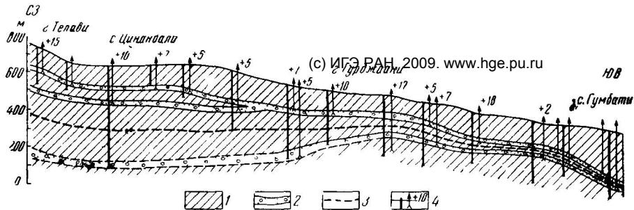
Рис. 17. Схематический гидрогеологический разрез по простиранию Телавского и Гурджаанского водоносных горизонтов (составили И. М. Буачидзе и С. Н. Зедгинидзе). 1—относительно водоупорные породы акчагыл-апшерона; 2—водоносные слои; 3—условная граница между Телавским и Гурджаанским горизонтами; 4—напор воды над устьем скважины
