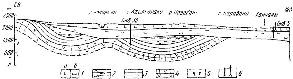
Рис. 16 Схематический гидрогеологический разрез Ахалкалакского лавового нагорья (составил Т. Х. Лазарашвили)
