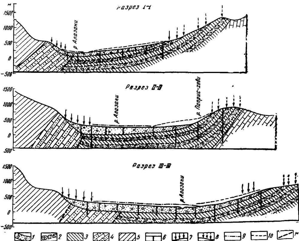
Рис. 14. Схематические гидрогеологические разрезы Алазанского артезианского бассейна (составили И. М. Буачидзе и С. Н. Зедгинидзе)
