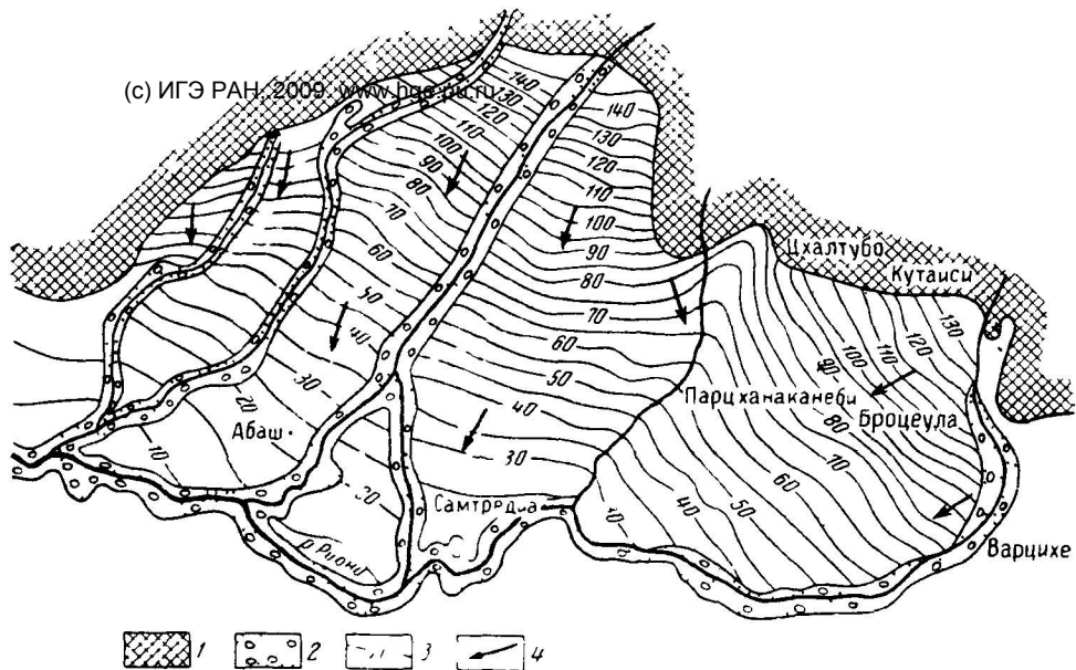
Рис. 9. Схематическая карта гидрогеогипс подземных вод древнечетвертичных отложений низменной части междуречья Риони—Техури (составил Л. А. Харатишвили) 1 — дочетвертичные породы; 2 — современный аллювий, 3 — гидрогеогипсы с абсолютной отметкой (в м), 4 — направление движения подземных вод.
