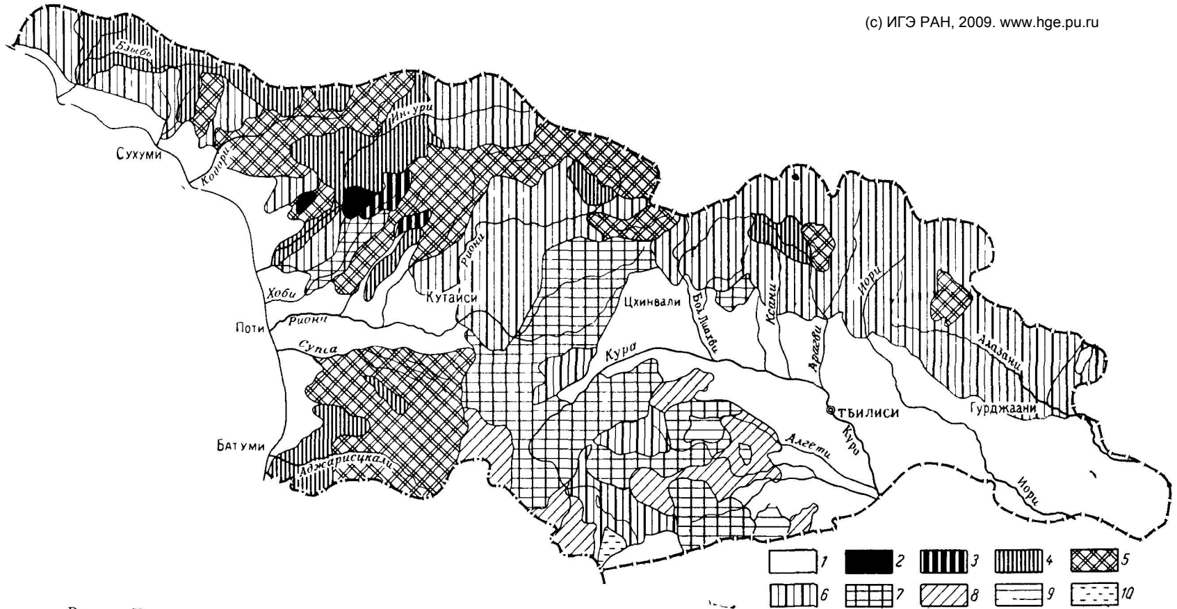
Рис 4 Карта подземного стока в реки Грузии (составили Л. А. Владимиров, Т. Н. Габричидзе, Д. И. Шакаришвили, Р. Г. Шенгелия) 1—более 1000 мм, 2—800—1000 мм, 3—600—800 мм; 4—400—600 мм; 5—200—400 мм; 6—100—200 мм; 7—50—100 мм; 8—10—50 мм; 9—0—10 мм, 10—районы с меднорагивными системами
