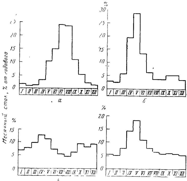
Рис. 3. Гидрографы рек с преобладанием ледникового (а), снегового (б), дождевого (в) и подземного (г) питания (составил Л. А. Владимиров)
