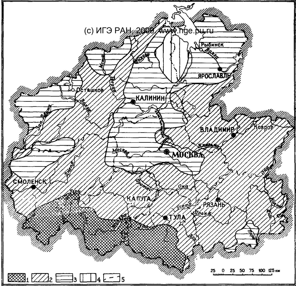
Рис. 46. Схематическая карта среднегогодового подземного стока в процентах от величины общего речного стока. Составила Н. А. Лебедева Величина подземного стока в реки (в % от величины общего стока рек) 1 — 50—40, 2 — 40—30; 3 — 30—20, 4 — <20, 5 — граница административных областей
