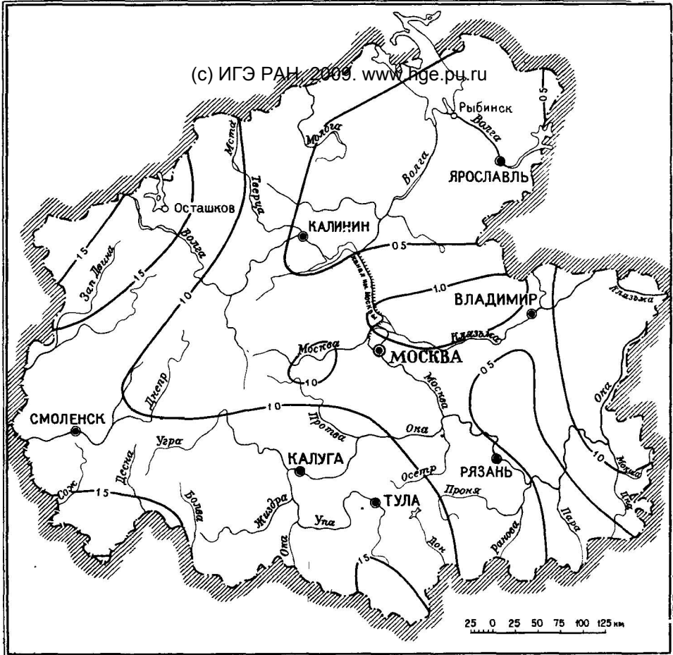
Рис. 45. Схематическая карта среднемноголетних минимальных природных ресурсов подземных вод в минимальных модулях подземного стока ( л/сек с 1 км^2 ). Составила Н. А. Лебедева
