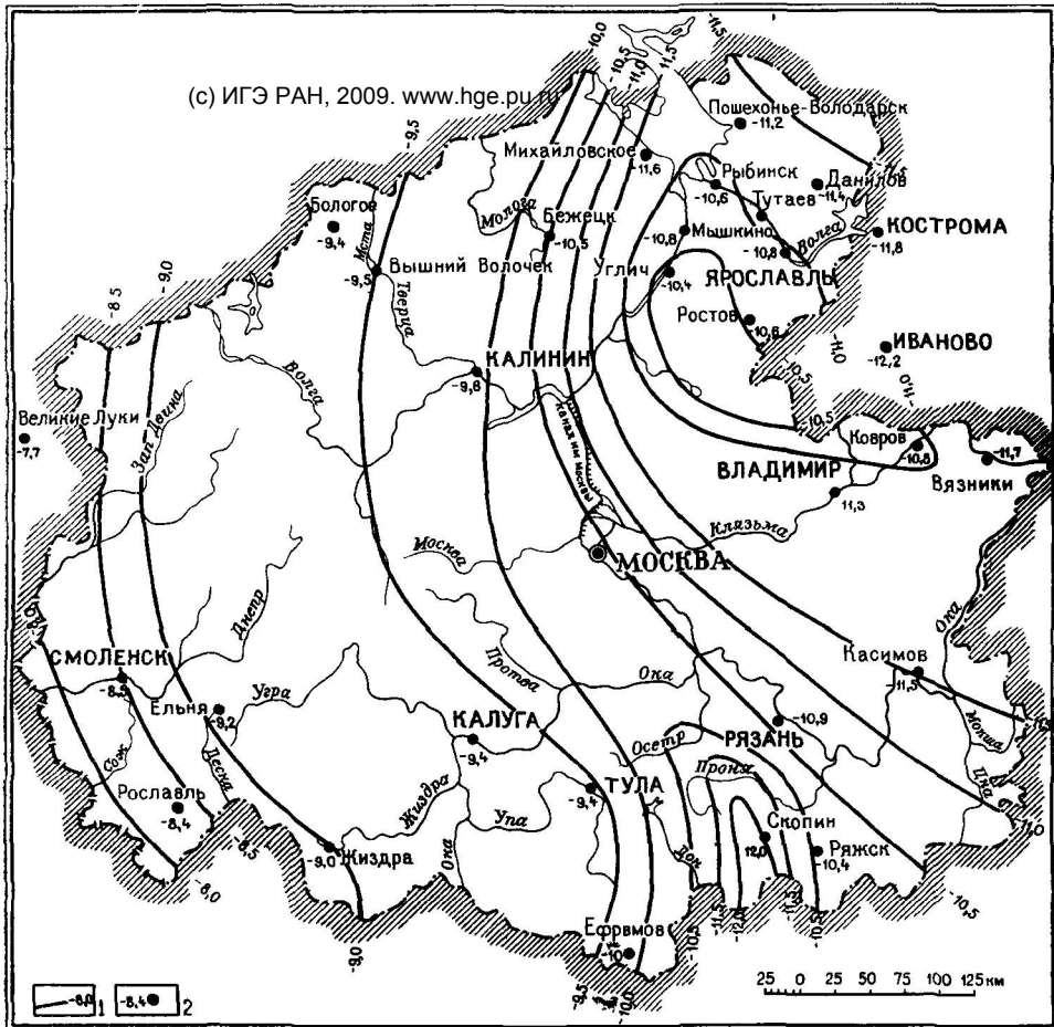
Рис. 4. Схематическая карта изотерм января. Составила Н. А. Молгачева по материалам Управления гидрометслужбы центральных областей 1 — изотермы января, 2 — средняя температура января в данном пункте
