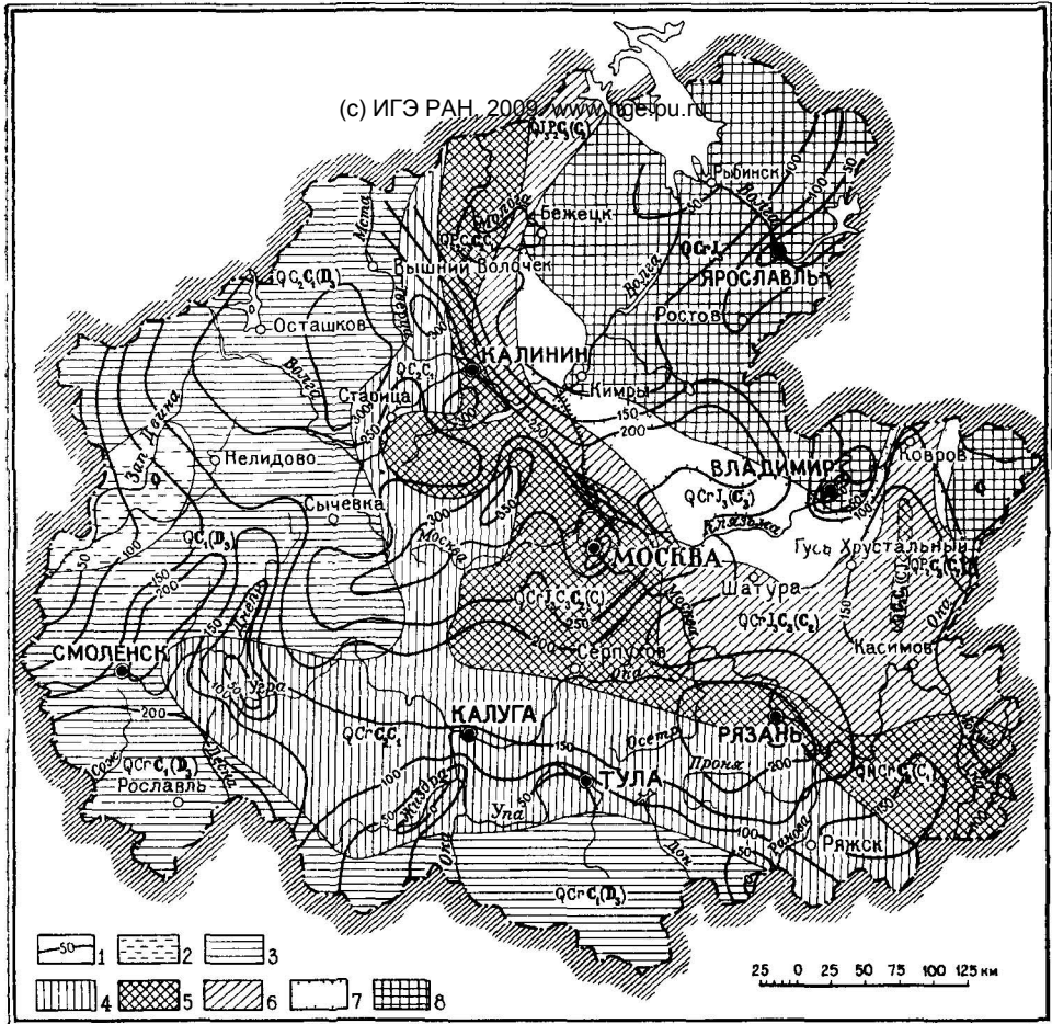
Рис 37 Карта глубин подошвы пресных вод Составила Н А Лебедева по материалам ГУЦР
