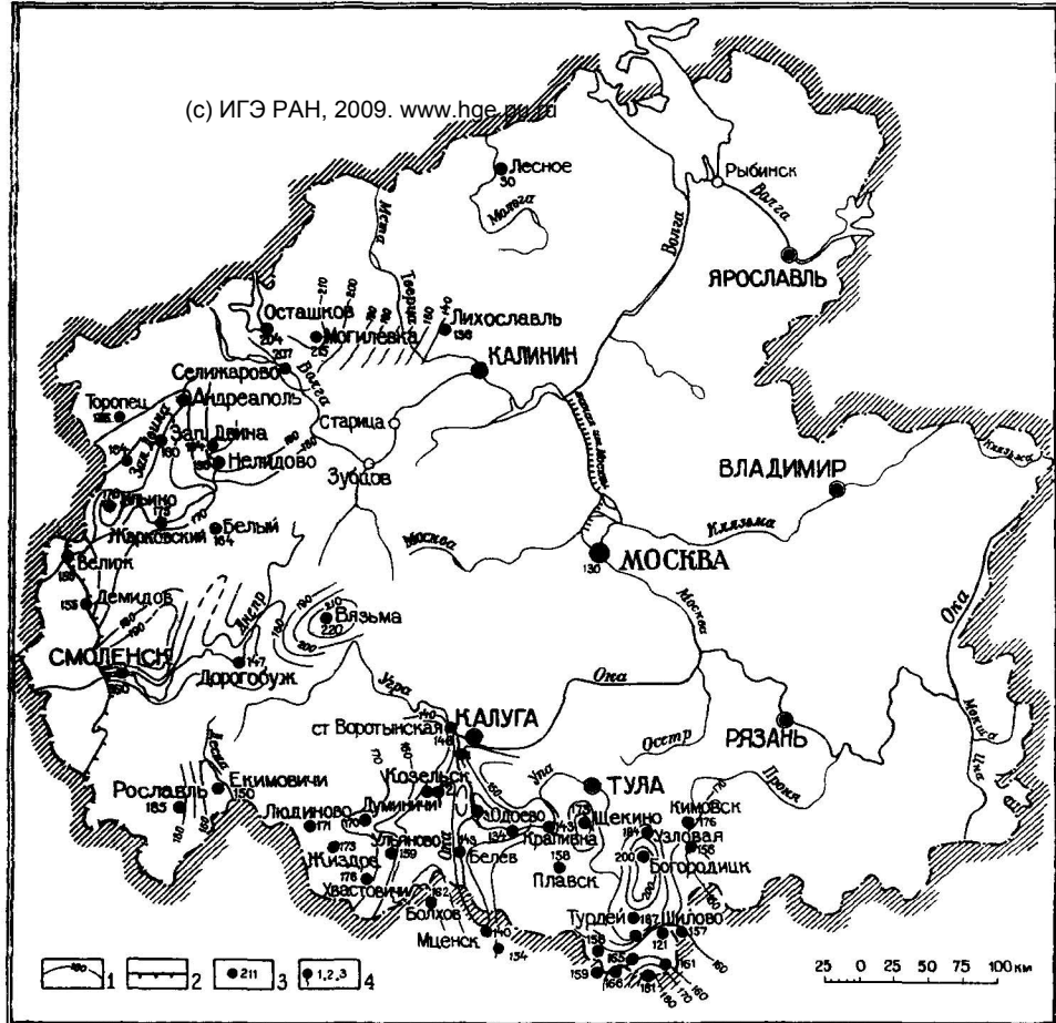
Рис. 30. Схематическая карта изопьез верхнефаменского D_3^{fm} водоносного комплекса. Составила Л. И. Флерова
