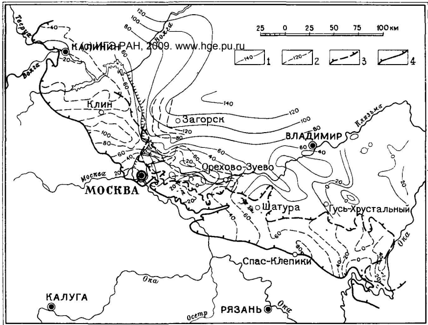
Рис. 24. Карта напоров над кровлей верхнекаменноугольных водоносных горизонтов (по материалам Подмосковной партии Гидрорежимной экспедиции ВСЕГИНГЕО, 1962 г)
