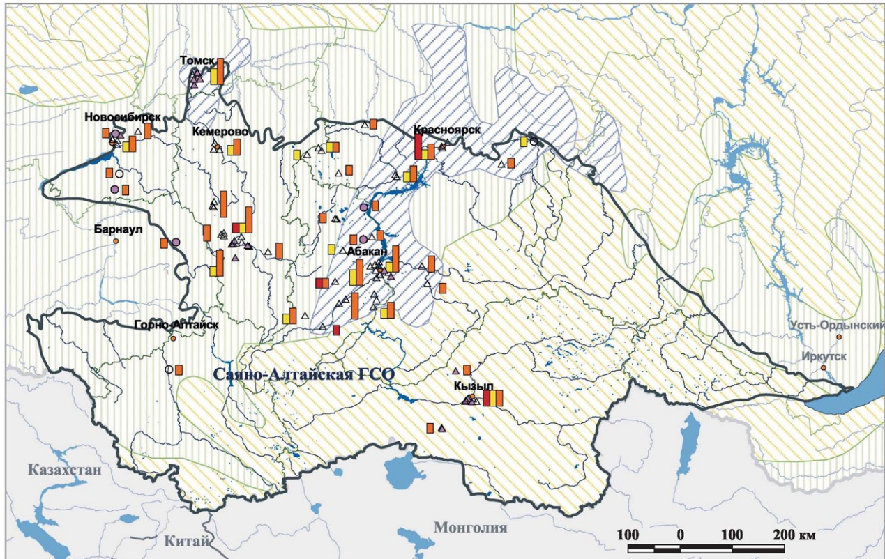
Рис. 1.45. Схема выявленных участков загрязнения подземных вод по классам опасности загрязняющего вещества на территории Саяно-Алтайской гидрогеологической складчатой области (по состоянию на 01.01.2008 г.)
