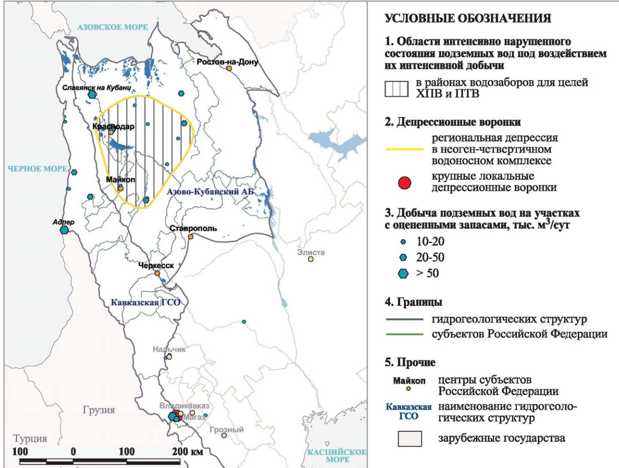
Рис. 1.28. Области интенсивно нарушенного состояния подземных вод на территории Азово-Кубанского артезианского бассейна и Кавказской гидрогеологической складчатой области (по состоянию на 01.01.2008 г.)
