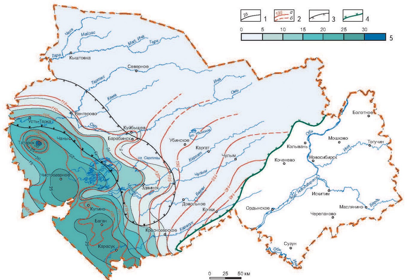
Рис. 1.29. Гидродинамическая карта подземных вод ниже-верхнемелового комплекса на территории Новосибирской области
