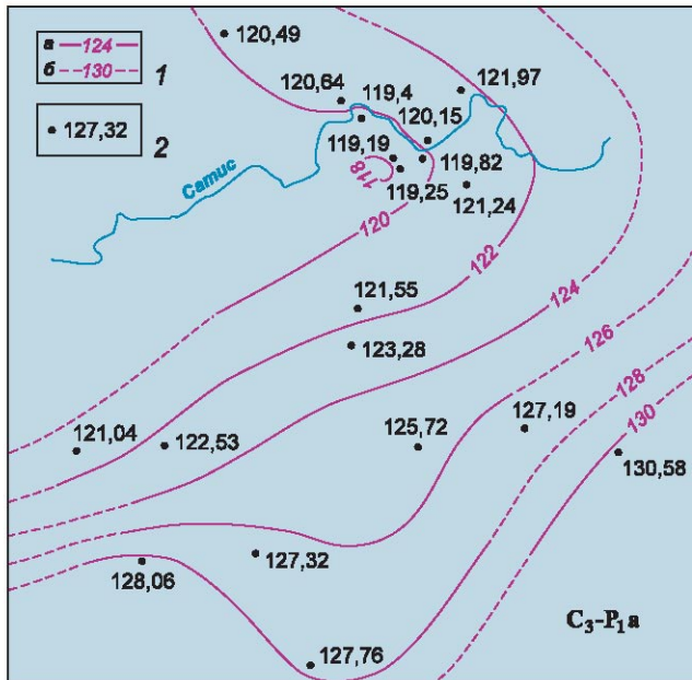
Рис. 1.24. Карта пьезоизогипс водоносной верхнекаменноугольно-ассельской карбонатной серии (С-Р 1 а) г.Сарова (Филипп ФГУГП "Волгагеология" Приволжский РЦ ГМСН)
