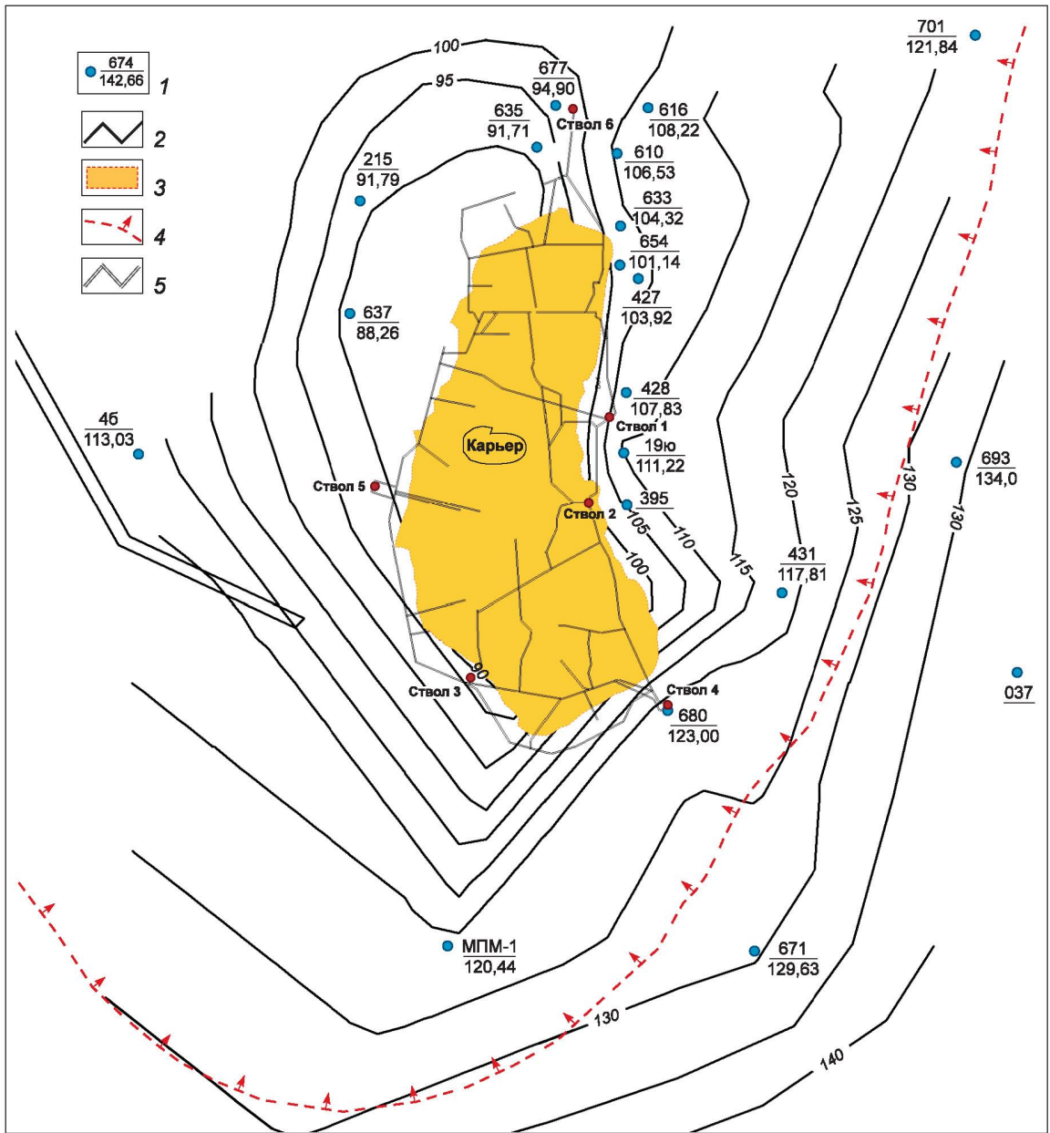
Рис. 1.41. Карта современного состояния подземных вод бат-кеповейского водоносного горизонта на территории Михайловского горно-промышленного района (Филиал ФГУП "Геоцентр-Москва" ТЦ ГМСН и ВО "Курсгеомониторинг"). Карта составлена режимной группой ОАО "Михайловский ГОК")
