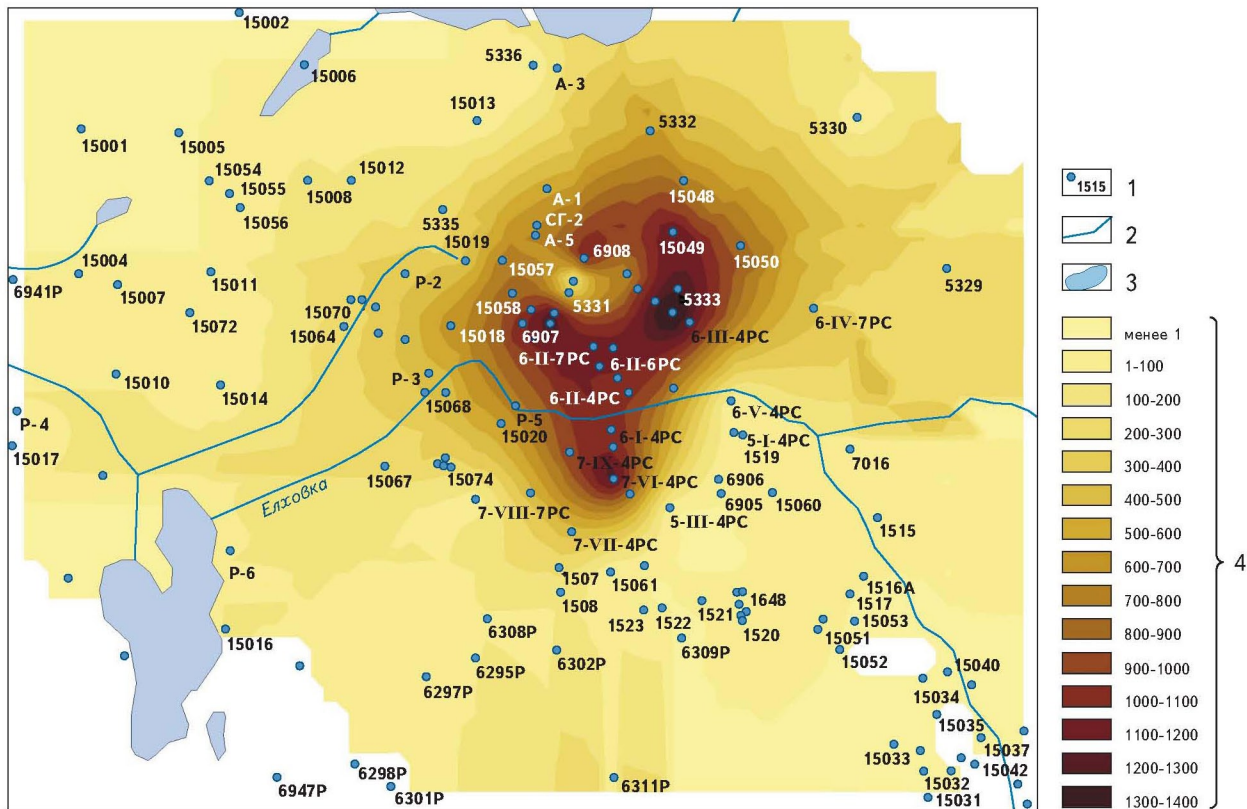
Рис. 1.51. Схема распространения нитратов в грунтовых водах полигона Кирово-Чепецкого химкомбината (Кировская обл.)
