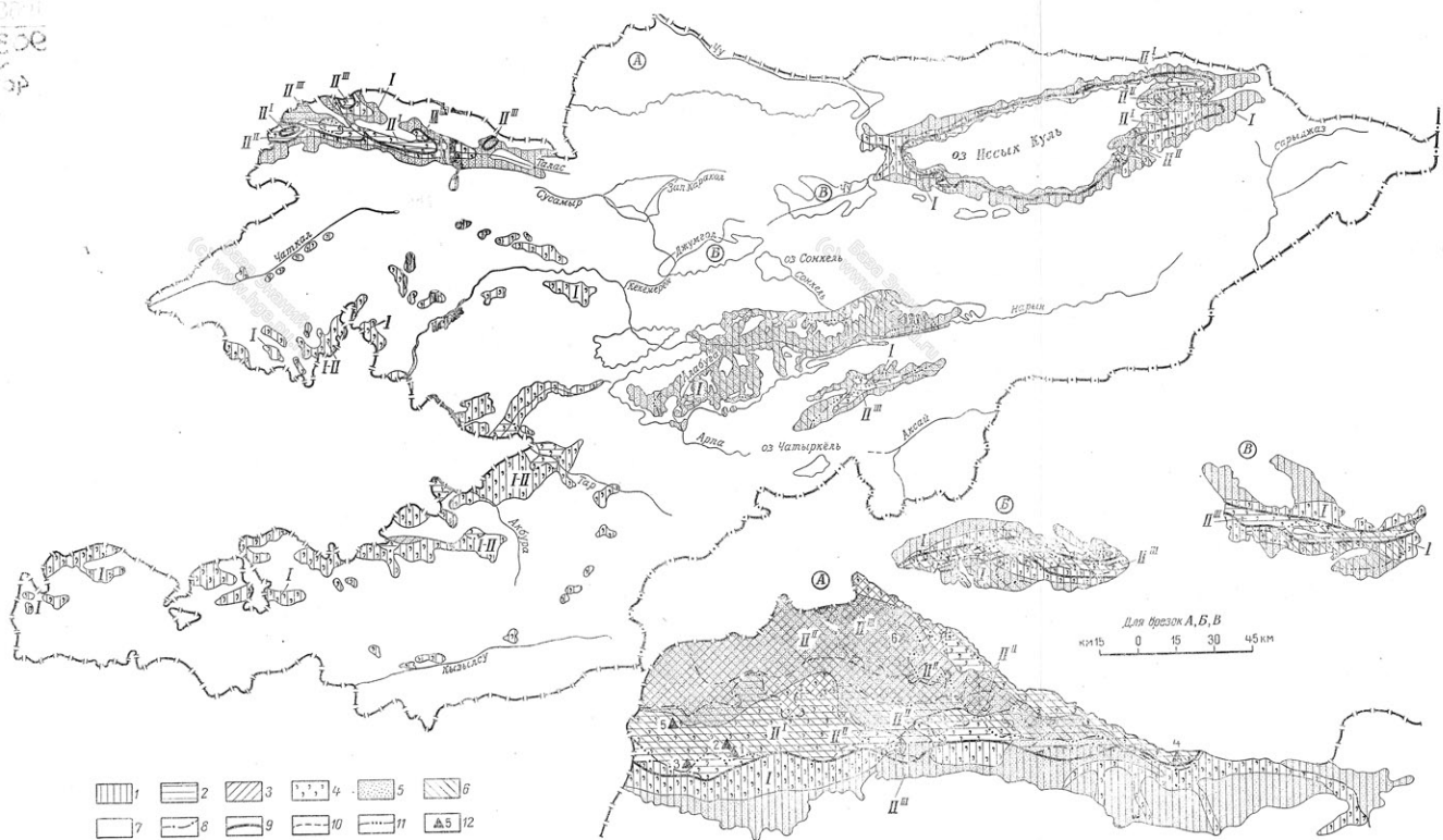
Рис. 37. Схематическая карта гидрогеологического районирования территории Карагандинской ССР по условиям применения вертикального дренажа (по Н. М. Каркищенко и Н. Г. Лютяевой, 1967). Зонам: 1 — интенсивно дренируемая; 2 — дренируемая; 3 — слабо дренируемая. Область: I — формирования грунтовых вод; II — формирования
