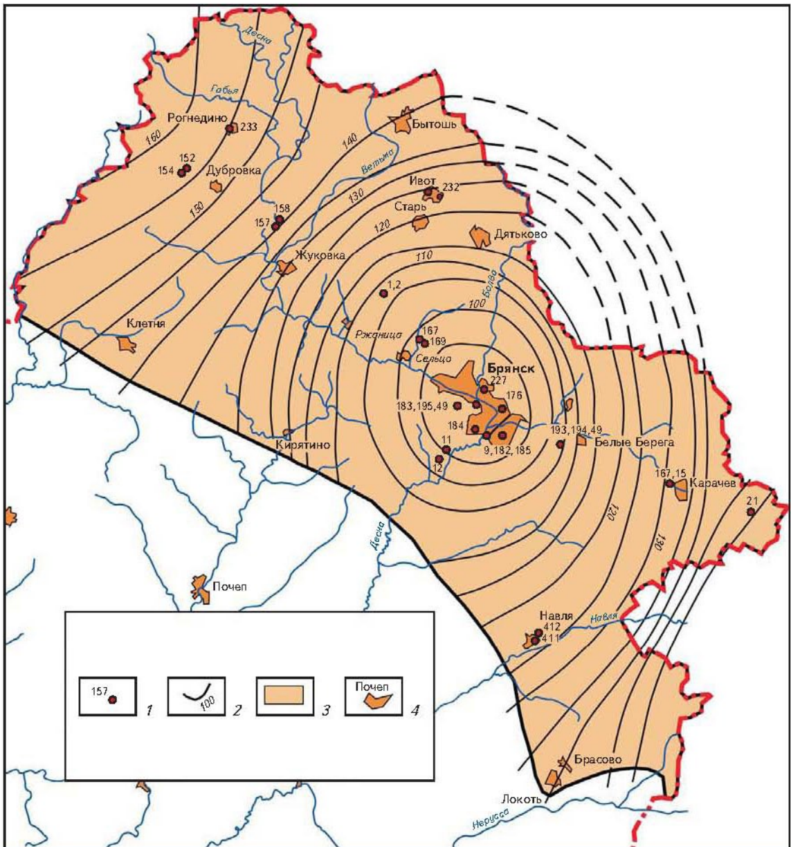
Рис. 1.15. Схематическая карта гидроизоэпез верхнефранско-фаменского водоносного горизонта на территории Брянской области (по данным Брянского ТЦ ГМСН, ФГУП "Геоцентр-Москва") 1 – наблюдательная скважина и ее номер; 2 – гидроизоэпеза и ее отметка; 3 – область распространения водоносной верхнефранско-фаменской терригенно-карбонатной свиты; 4 – населенные пункты
