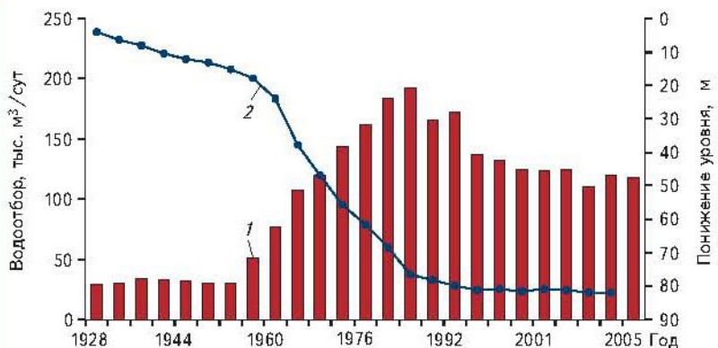
Рис. 1.16. Графики изменения водоотбора (1) и уровня (2) подземных вод верхнедевонских водоносных горизонтов (г.Брянск) (Брянский ТЦ ГМСН, ФГУП "Геоцентр-Москва")
